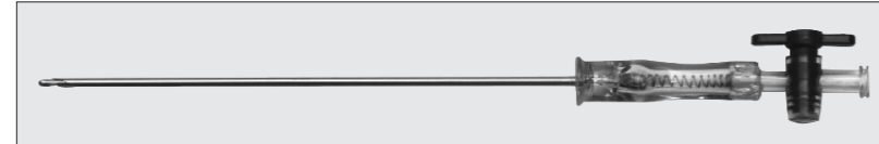
一次性使用气腹针 Disposable veress needle 701.004 \Phi 2.1mm
